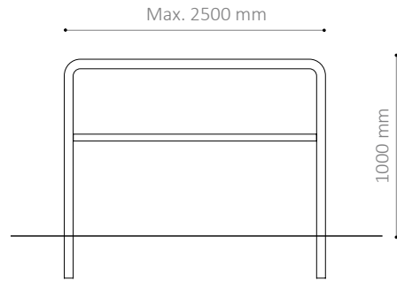
TYPE A3
